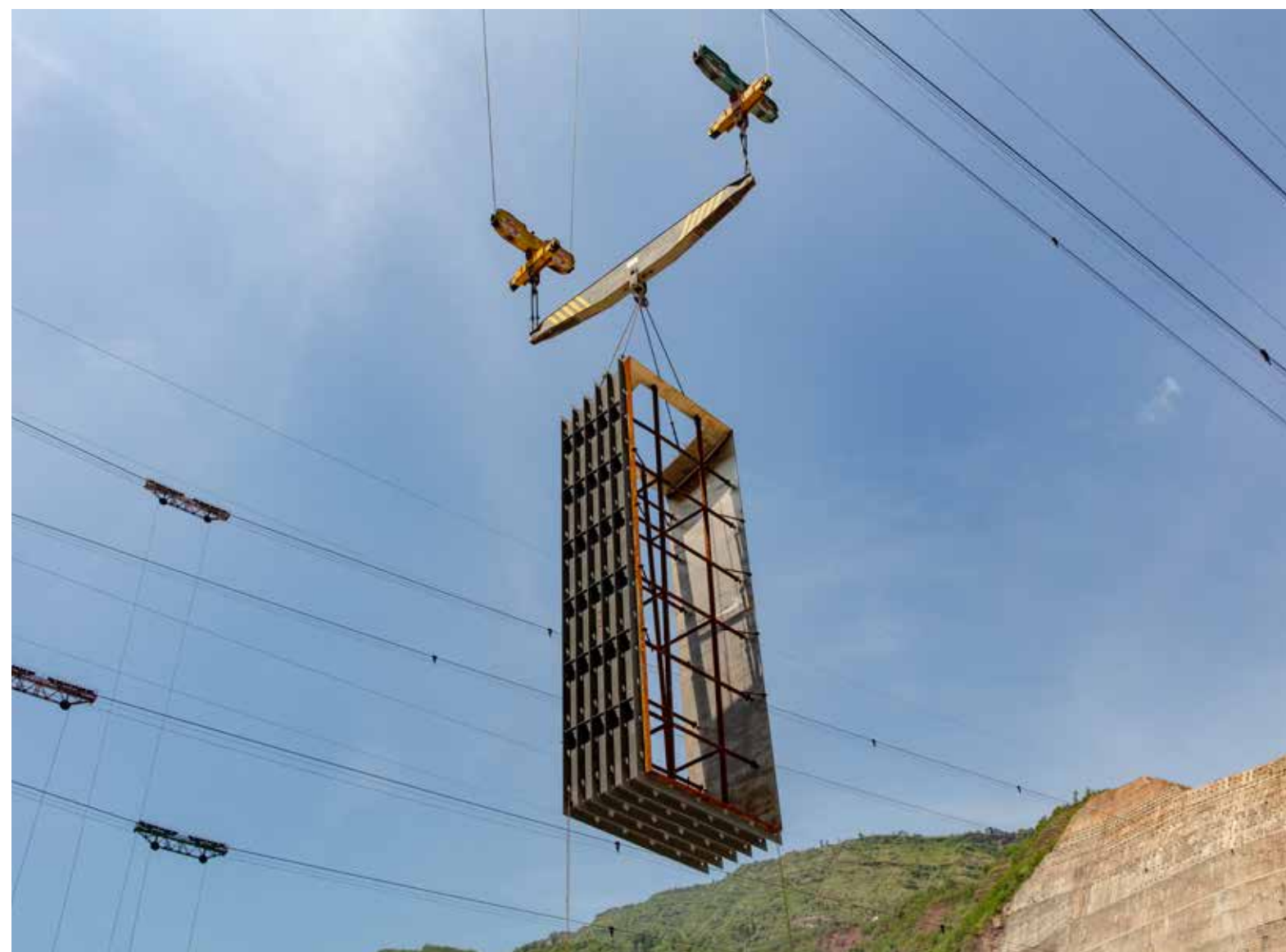
19 号坝段导流深孔钢衬吊装
