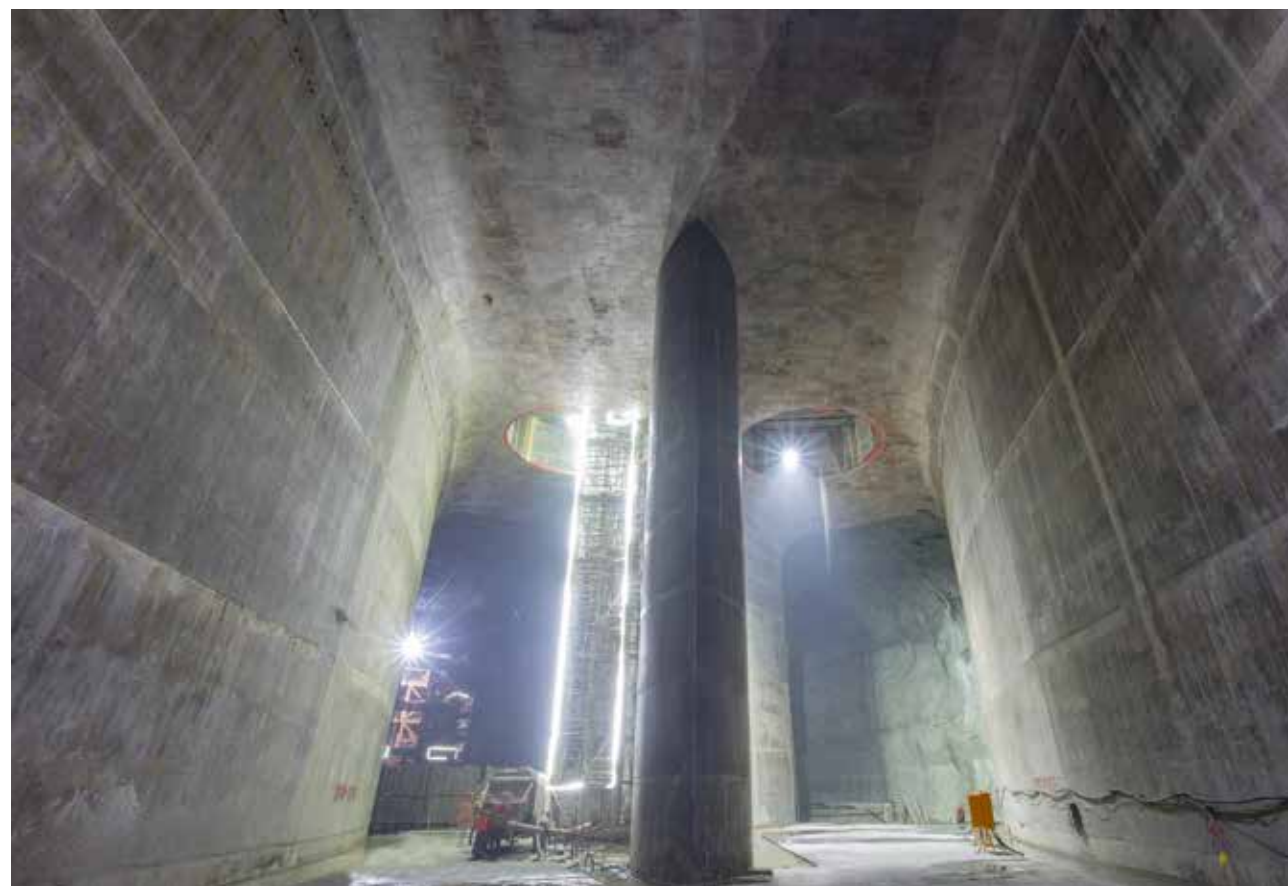
尾水调压室流道混凝土浇筑形象
