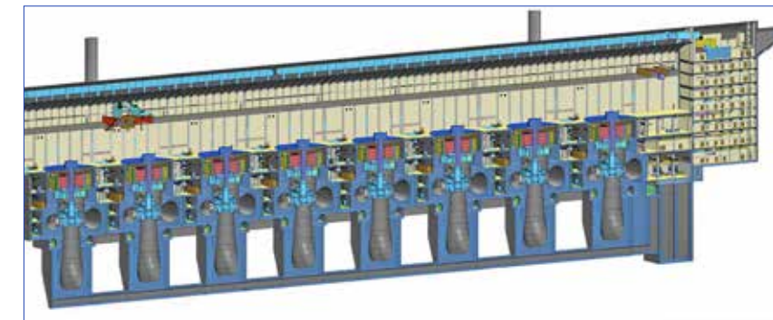
地下厂房纵剖面图
