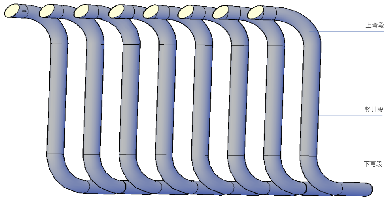
压力管道结构三维效果图
