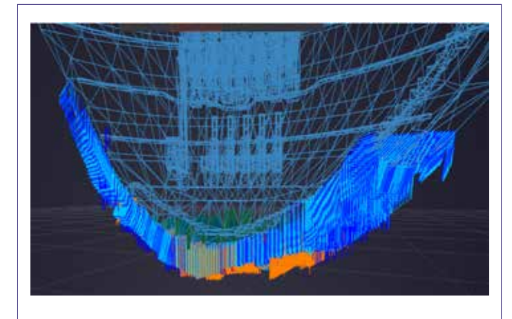
大坝三维地质与渗流模型
