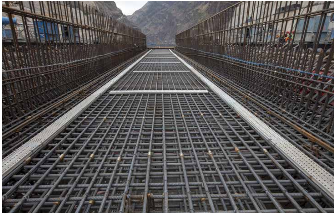
大坝导流孔底板钢筋备仓
