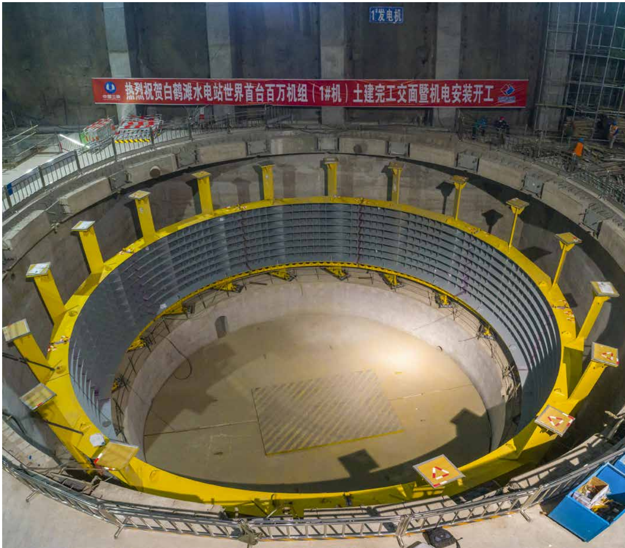
2019年左岸1号机窝施工形象
