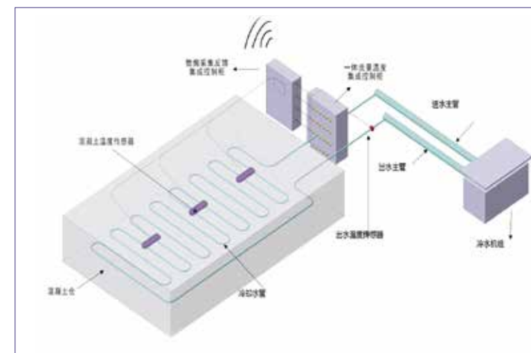
大坝混凝土智能通水系统
