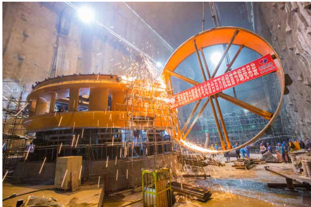
左岸1号机组首节蜗壳挂装
