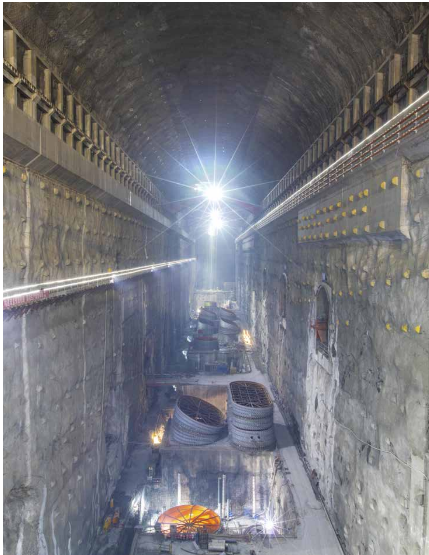
地下厂房肘管与锥管安装现场
