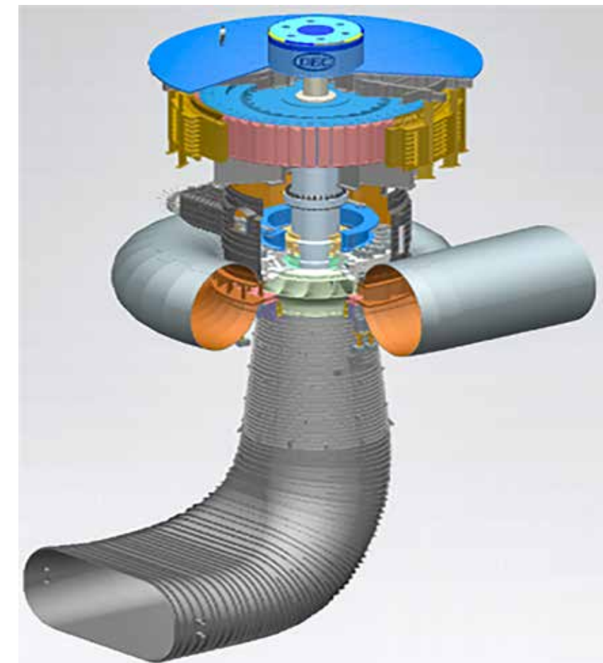
水轮机组三维效果图
