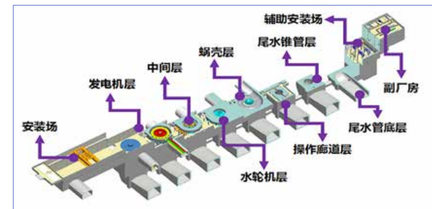
水轮机组结构布置示意图
