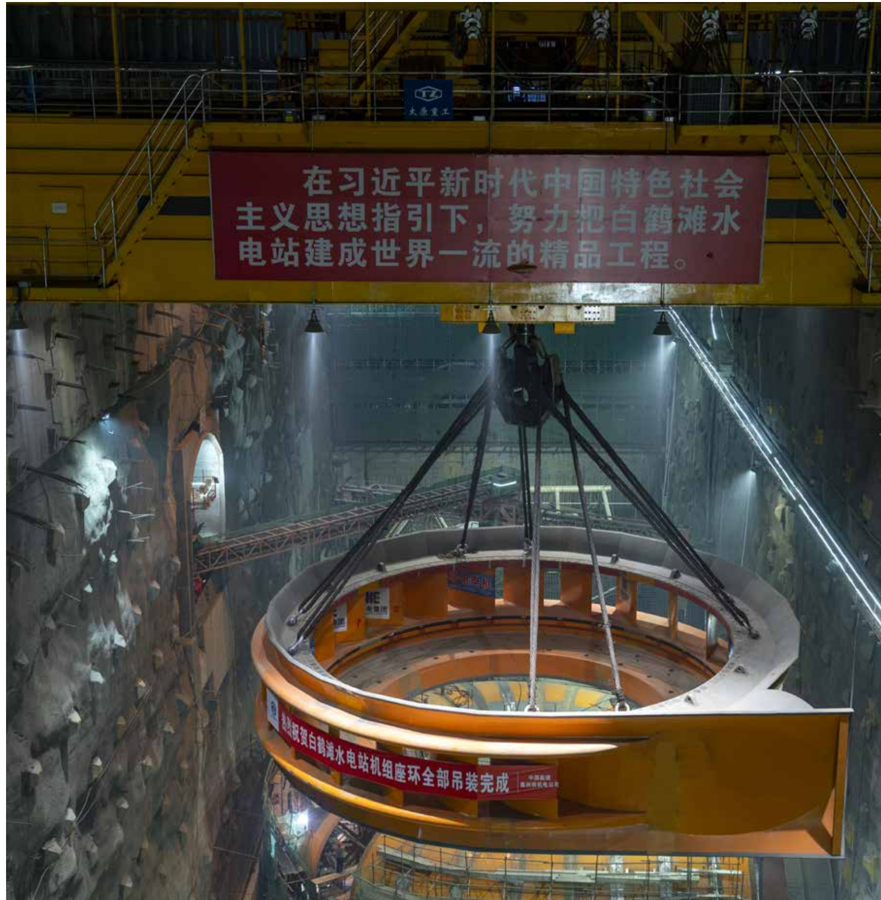
右岸最后一台座环圆满完成吊装
