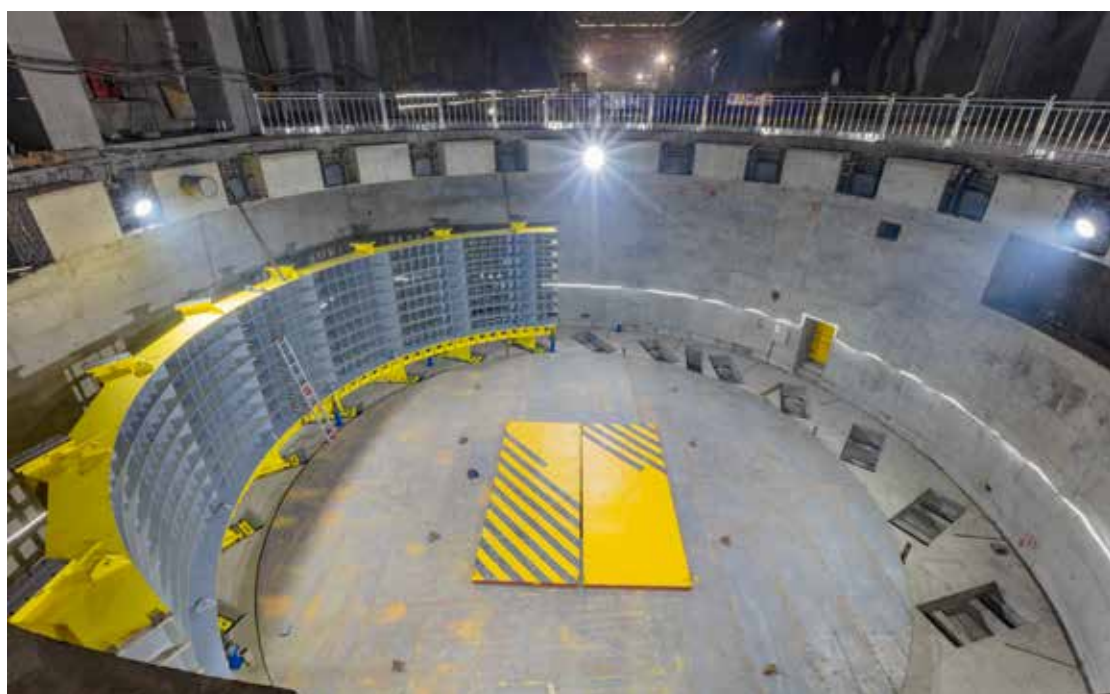
机组埋件安装形象
