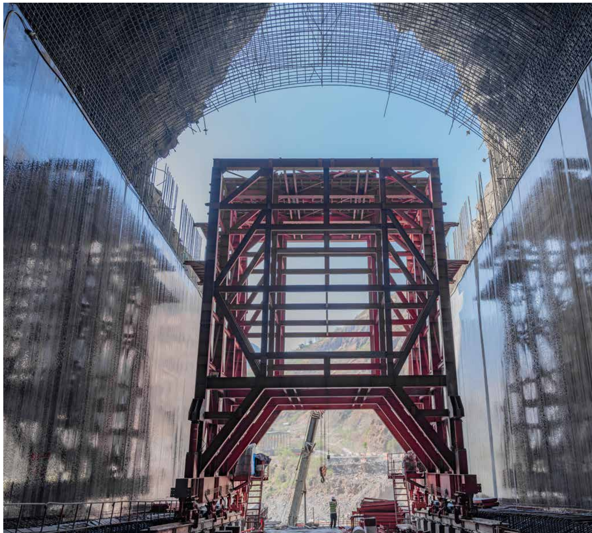
2019 年左岸 3 号泄洪洞龙落尾出口边墙衬砌施工形象
