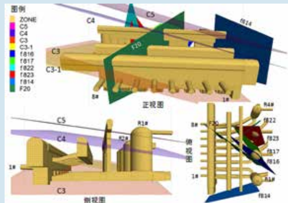
白鹤滩右岸地下厂房洞室群地质条件
