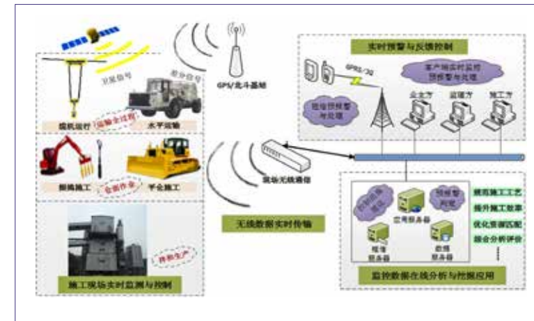
大坝混凝土浇筑“一条龙”全过程高效施工智能控制系统
