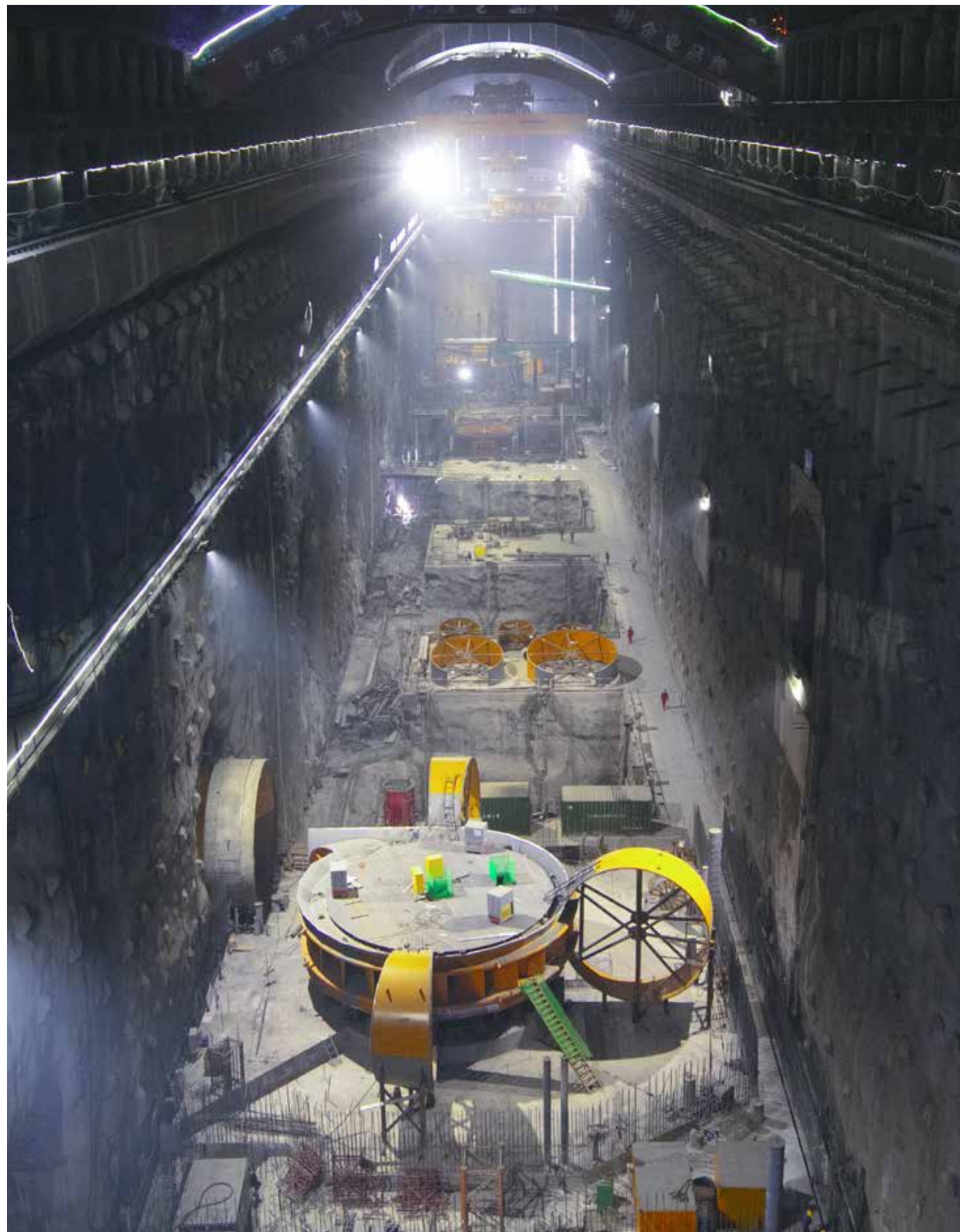
右岸主厂房安装施工形象
